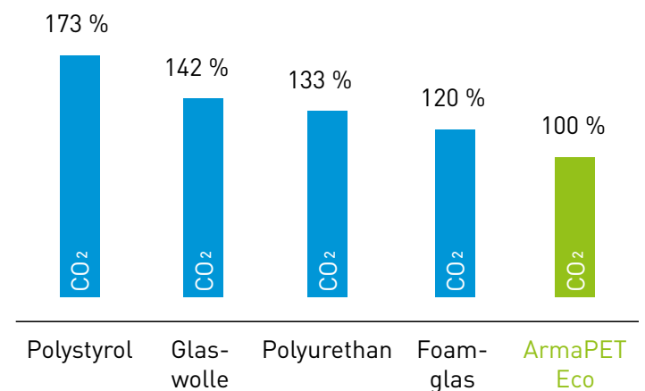
CO 2 -Emissionen von ArmaPET Produkten im Vergleich zu Wettbewerbsmaterialien. ArmaPET = 100 % Referenz.
